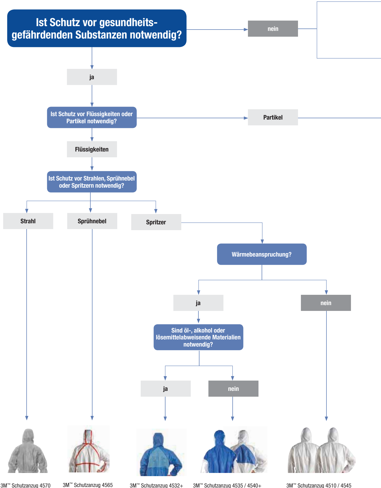
3M™ Schutzanzug 4570
